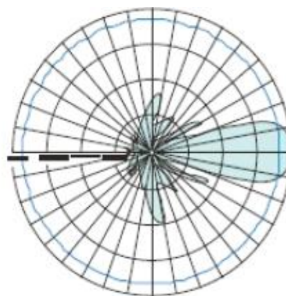
E-Plane
