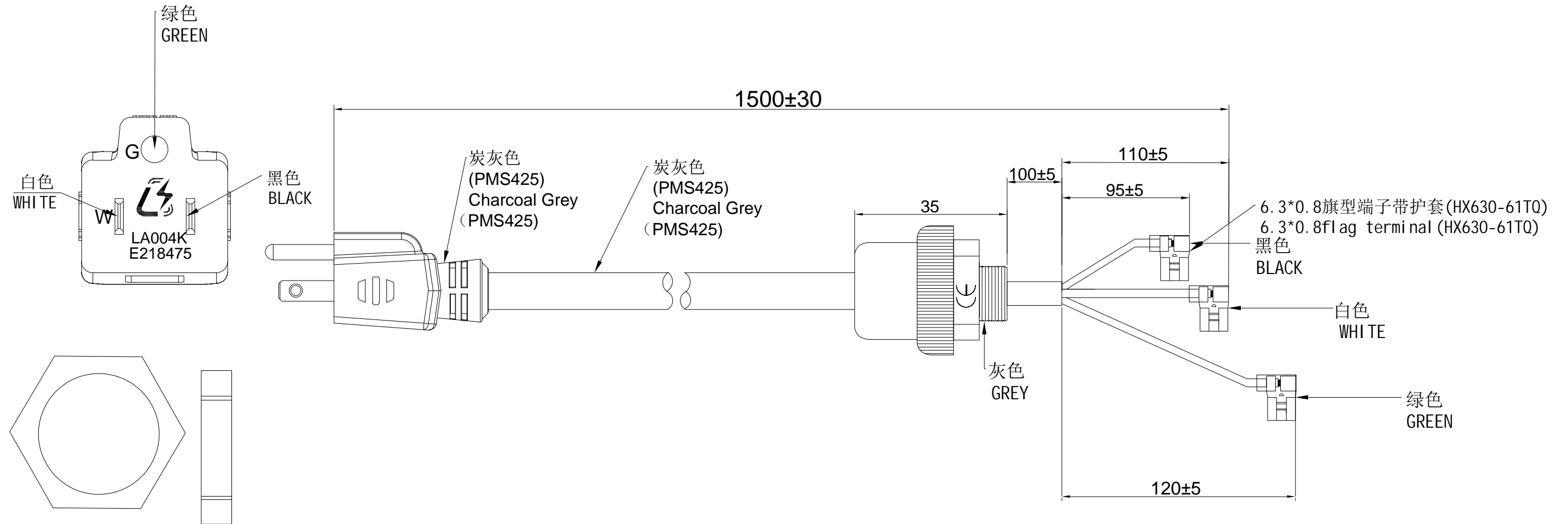
线扣螺帽示意图: Supply nut for cable gland diagram:
